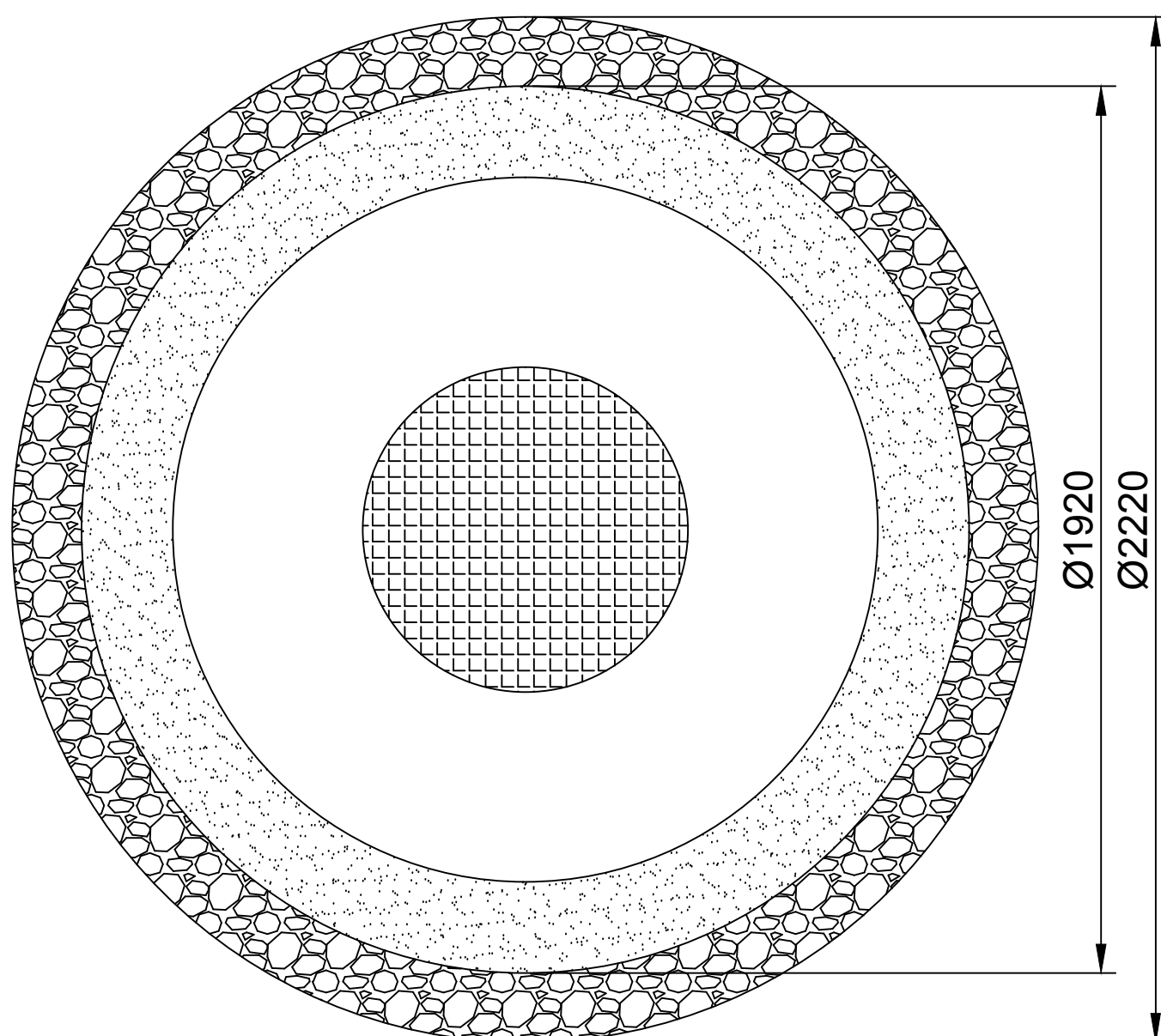
Монтажная схема ЛОС-8
