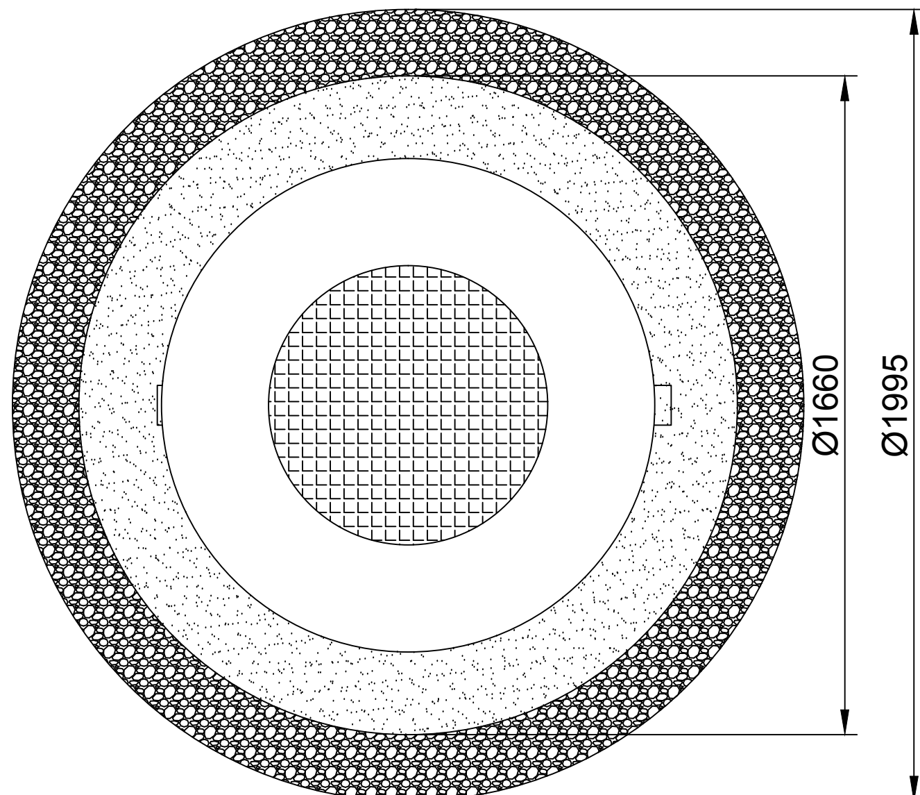
Монтажная схема ЛОС-5
