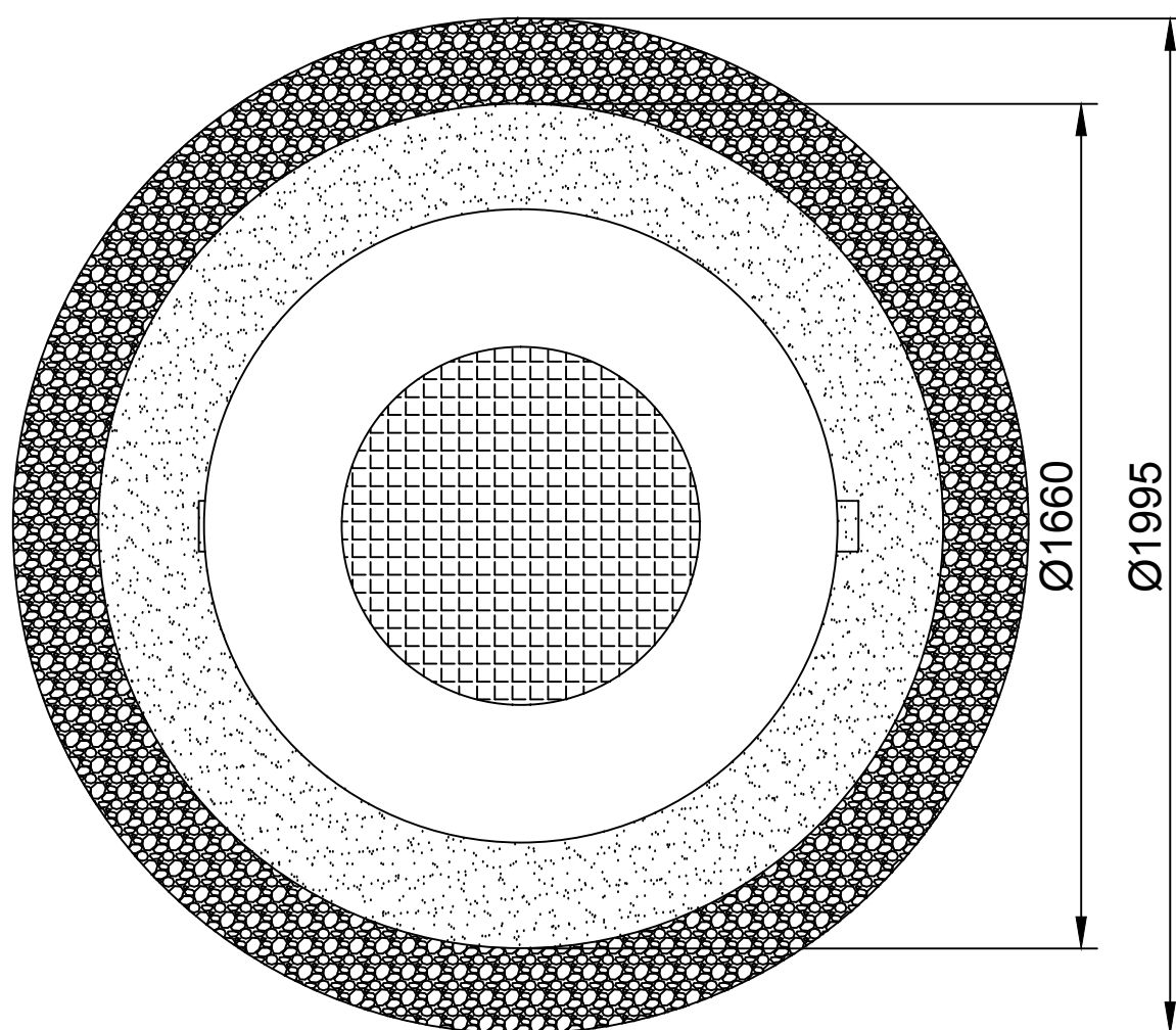
Монтажная схема ЛОС-5 Long
