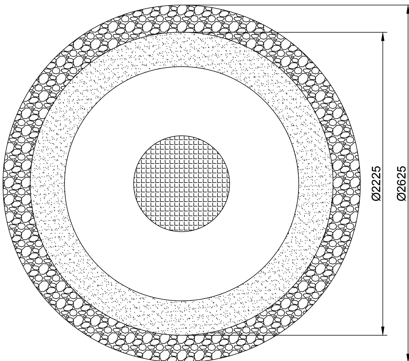
Монтажная схема ЛОС-15
