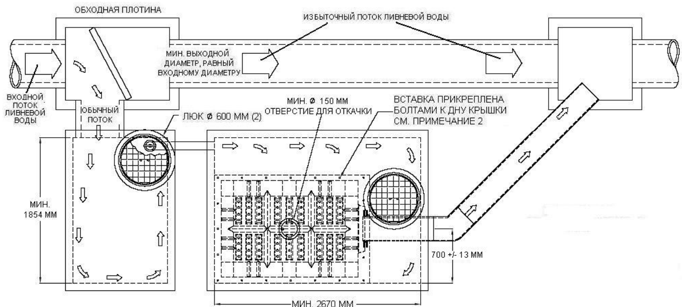
ВИД СВЕРХУ
