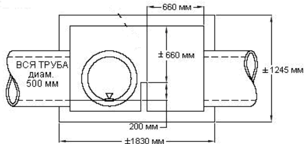
ВЕРТИКАЛЬНЫЙ РАЗРЕЗ МОДУЛЯ ПЛОТИНЫ
