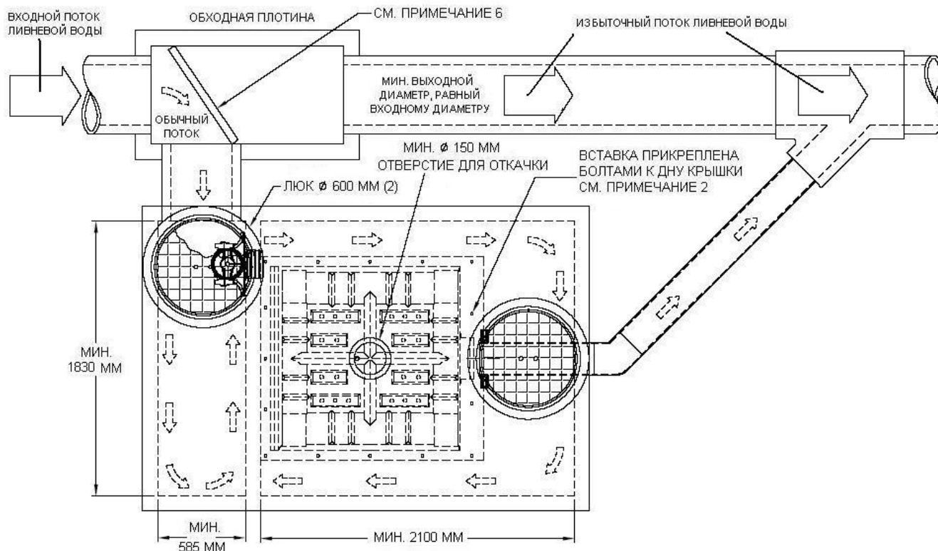
ВИД СВЕРХУ
