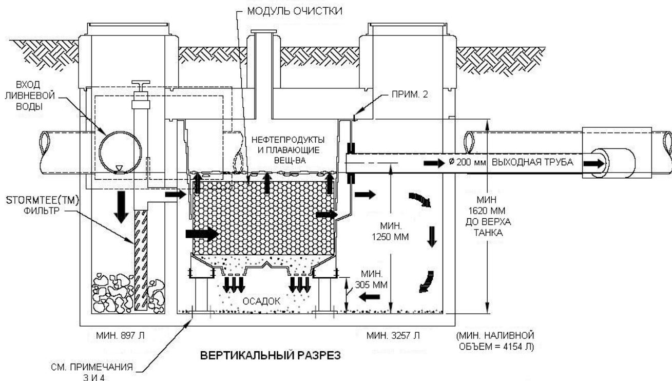
Рис.2. Общий вид системы очистки.
